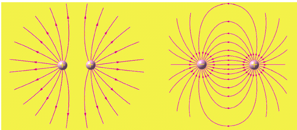
IMAGEN 58 A. Campo eléctrico producido por un conjunto de cargas puntuales. Se muestra en rosa la suma vectorial de los campos de las cargas individuales.
