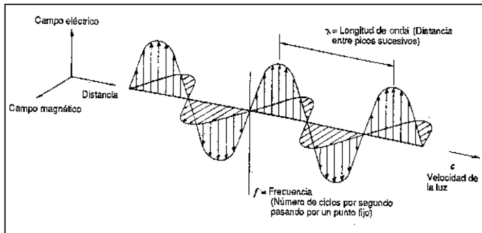
IMAGEN 56. Ondas electromagnéticas. (Licencias Creative Commons).
