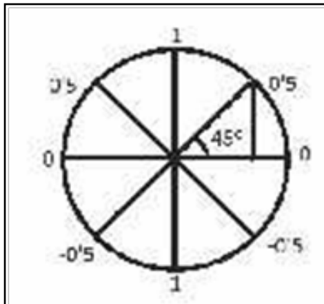
FIGURA 4. Con una simple calculadora, podemos ver el valor de los senos de distintos ángulos: el seno de 45° es 0,5; el de 90° es 1, etc. (Imagen del autor).
