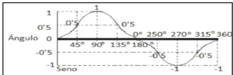
Figura 5. A cada ángulo (eje x) le corresponde un seno, un punto en la curva. Todos los puntos de la onda son senos de ángulos = \sin \alpha . (Imagen del autor).
