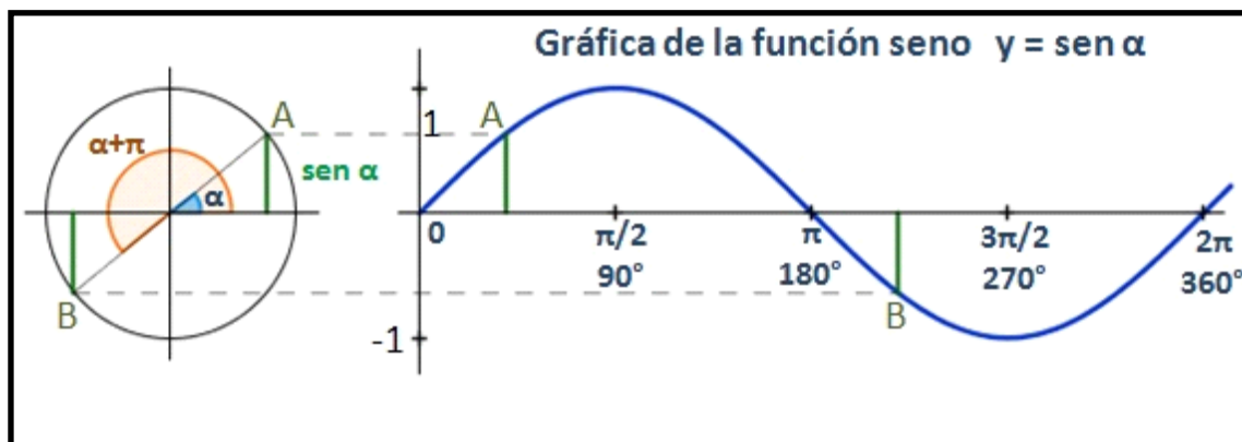
FIGURA 3. Basta mirar esta figura, para entender claramente que a cada seno (en verde) le corresponde un punto en la curva; todos los puntos de la curva son senos de un ángulo. Las ondas tienen pues un carácter angular. (Imagen autor desconocido. Autorizada Licencia Commons. Imágenes en línea, Word). IMAGEN 53
